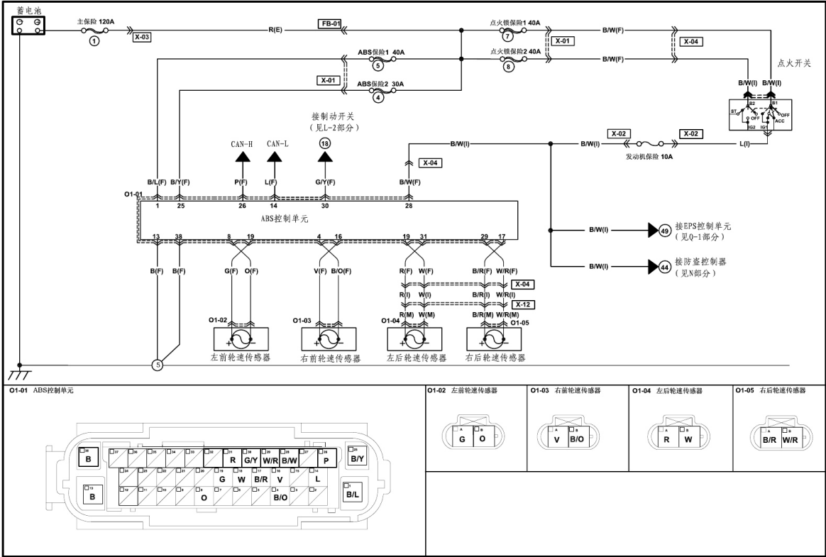
ABS系统
